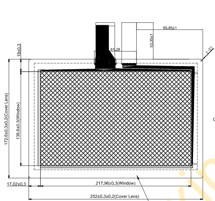
正視圖
