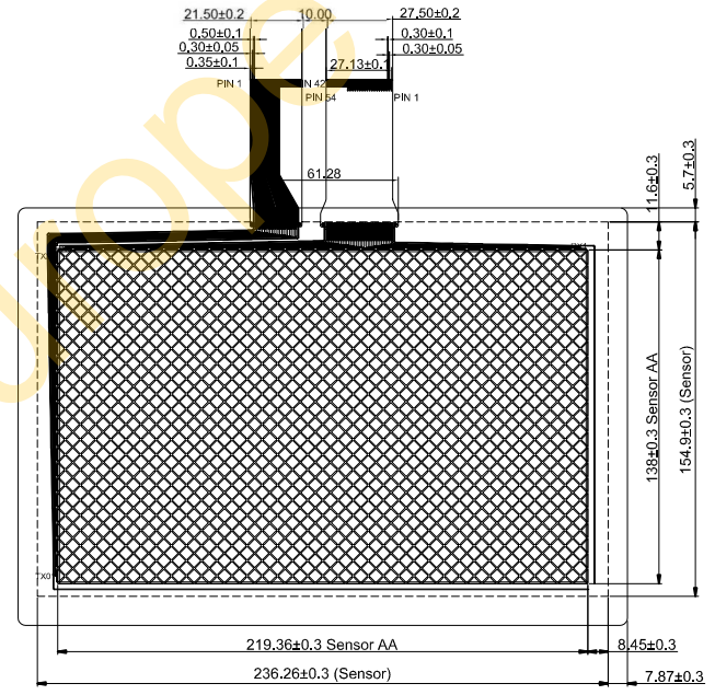
背視圖
