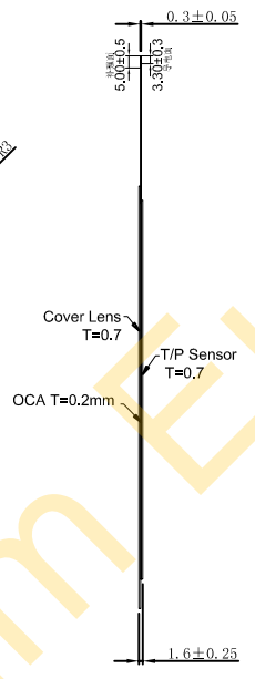
側視圖
